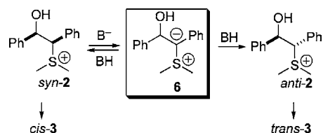
Scheme 4. Isomerization of syn -2 via C–H Deprotonation
